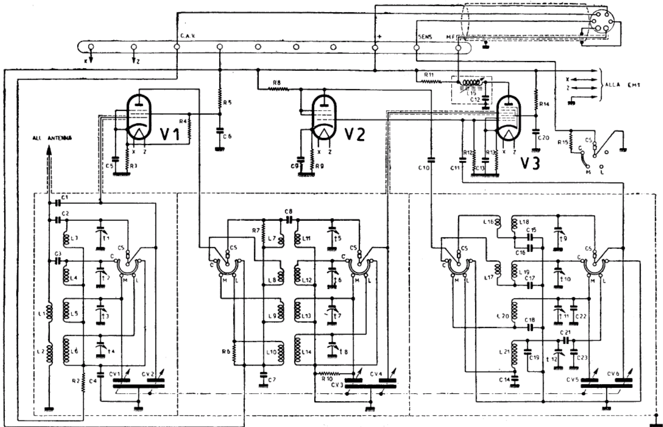
- Ricevitore supereterodina a 18 valvole.
